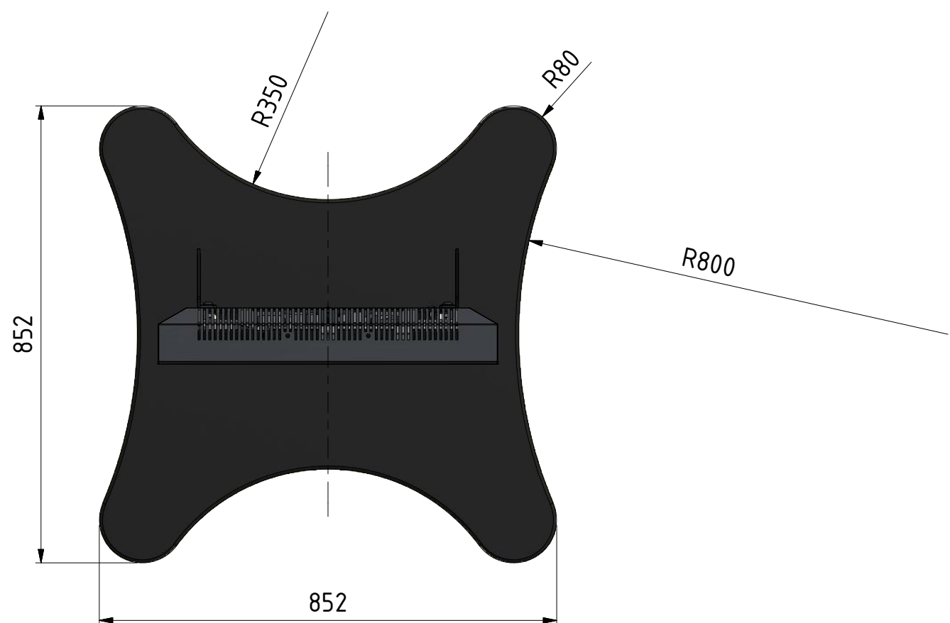
Ansicht von Oben / TOP VIEW
