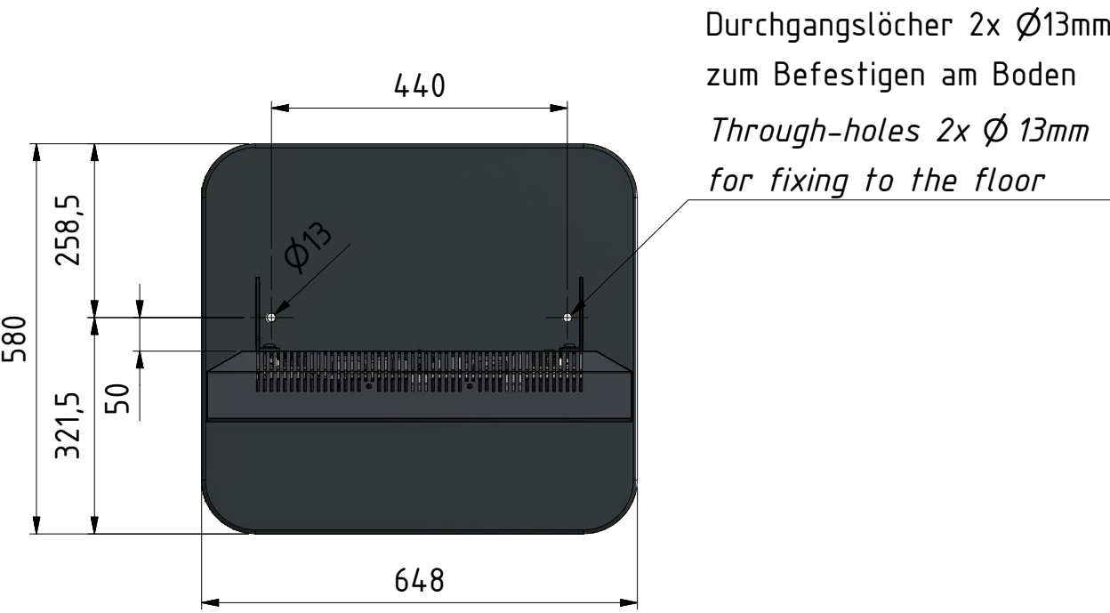
Ansicht von Oben / TOP VIEW
