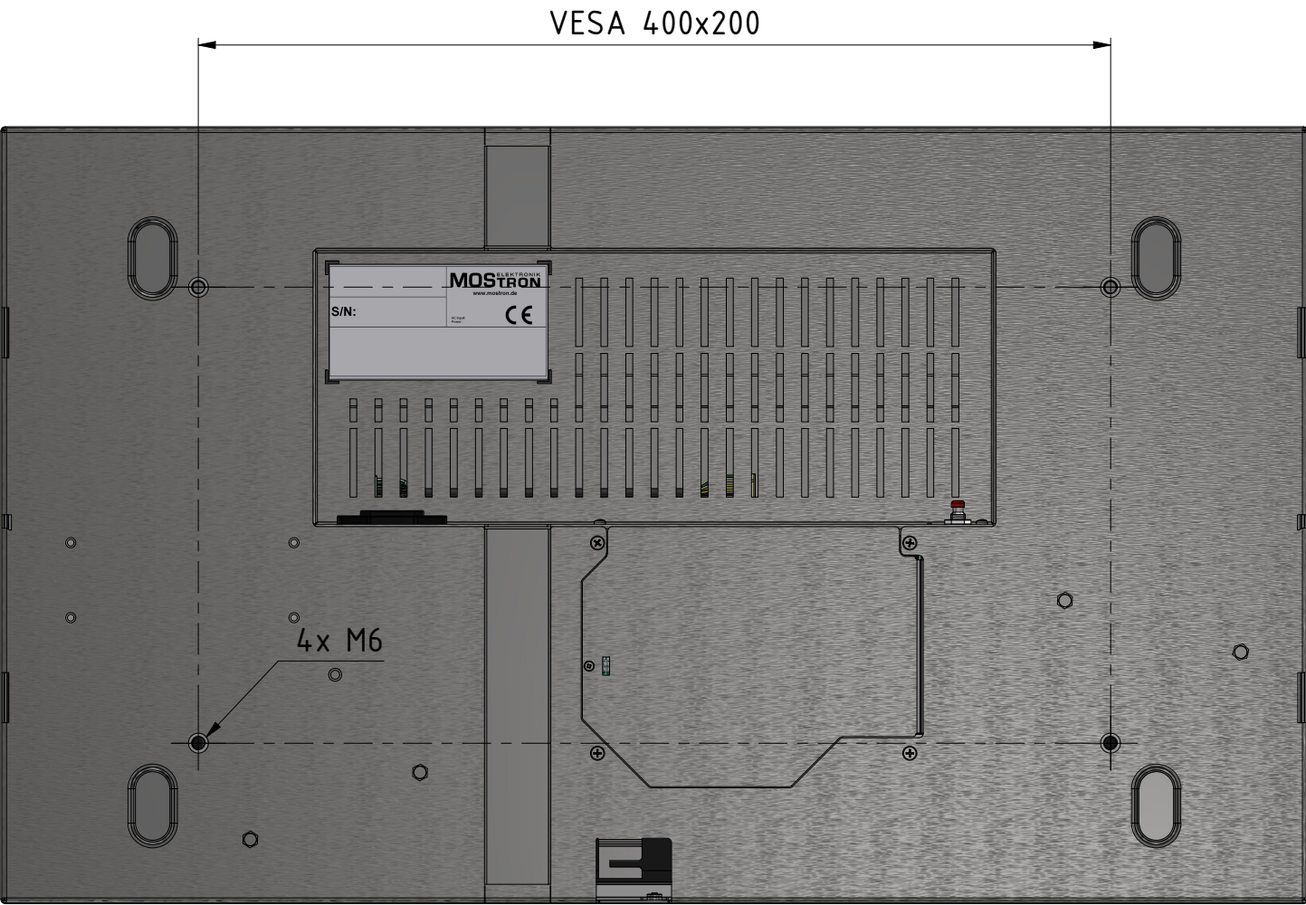
Rückansicht / BACK VIEW
