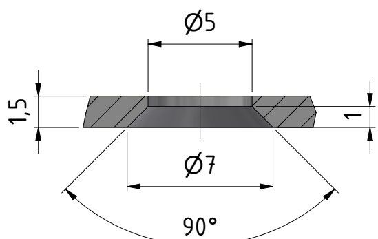
B-B ( 4 : 1 )
