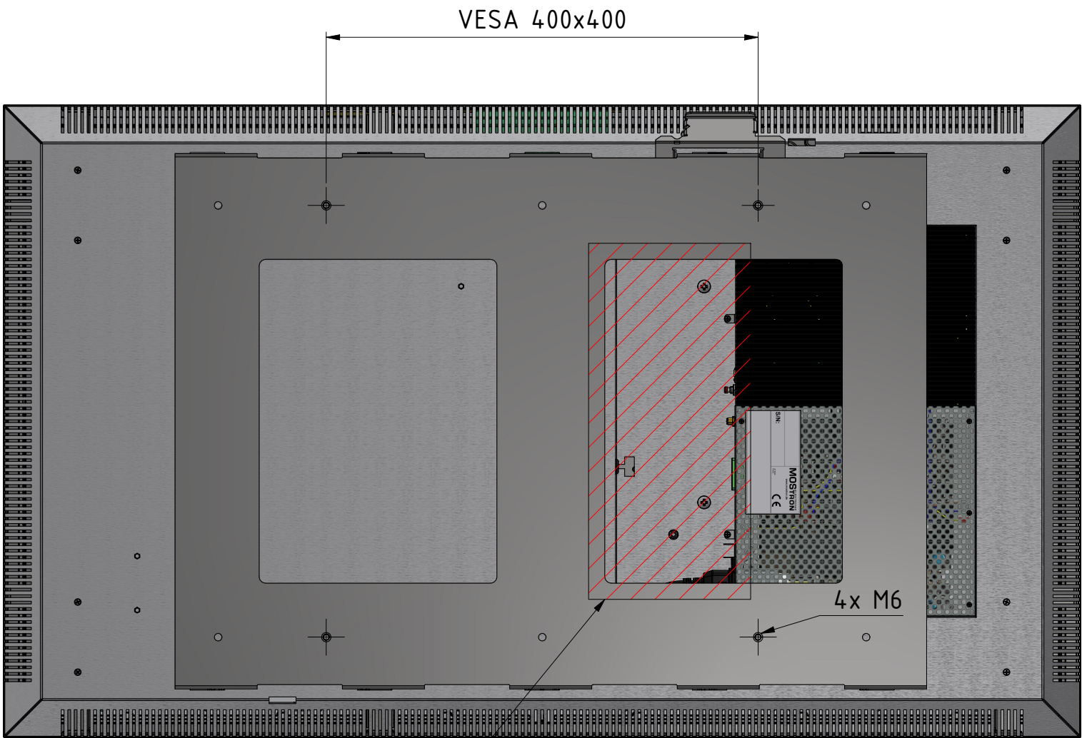
Bereich für Kabeldurchführung cable entry area
