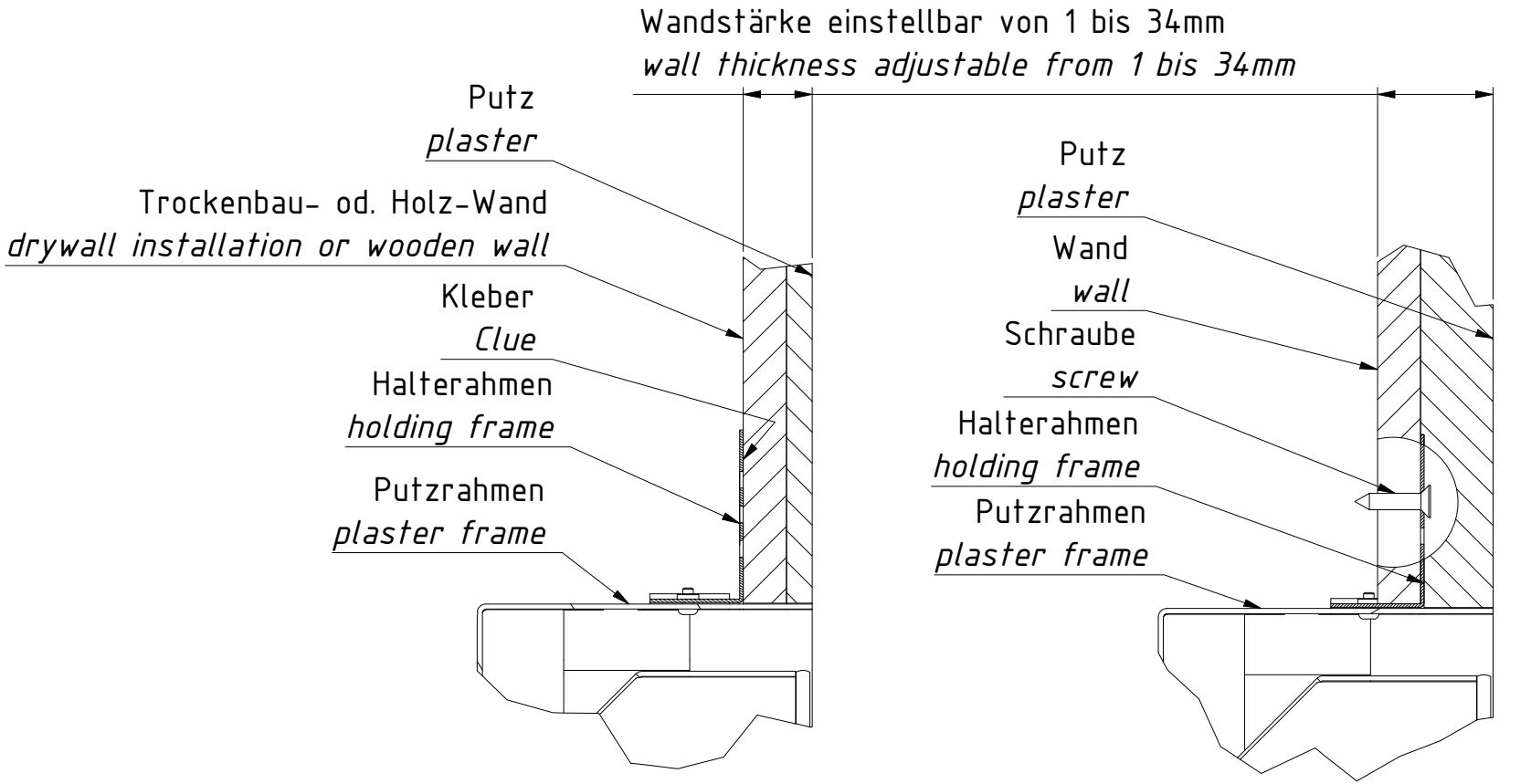
Montageart 'B' Assembly type 'B'
