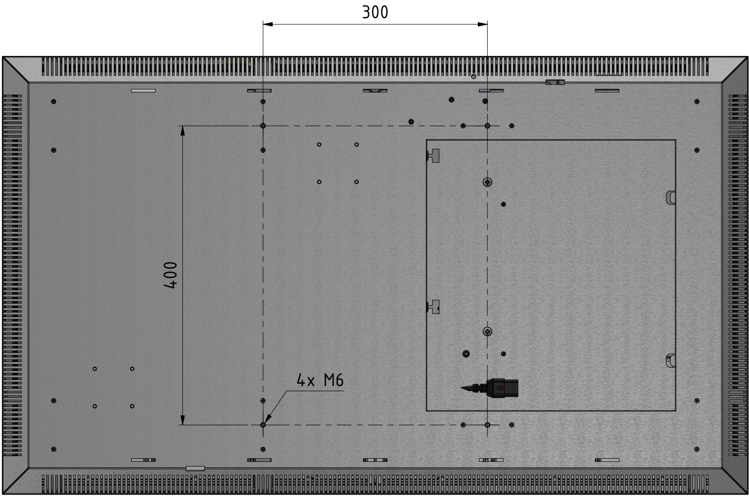
Rückansicht / BACK VIEW
